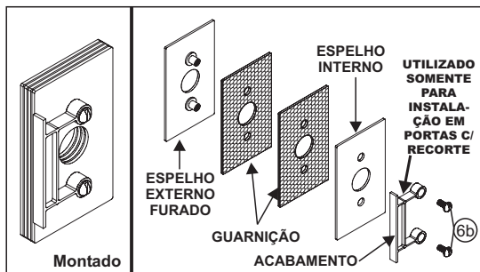
Figura 3 - Espelhos, guarnições e acabamento, para fixar a Fechadura.
